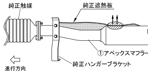
遮熱板加工指示詳細図
