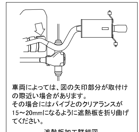
遮熱板加工詳細図
