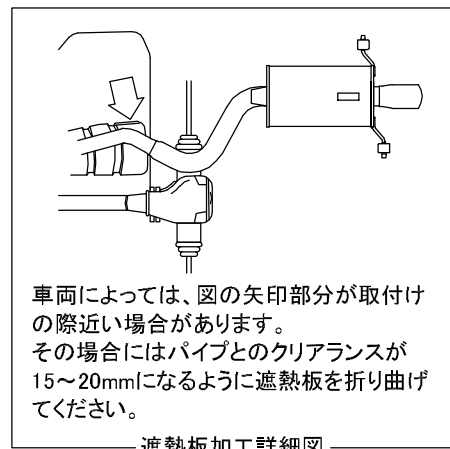
遮熱板加工詳細図
