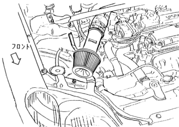
完成図
