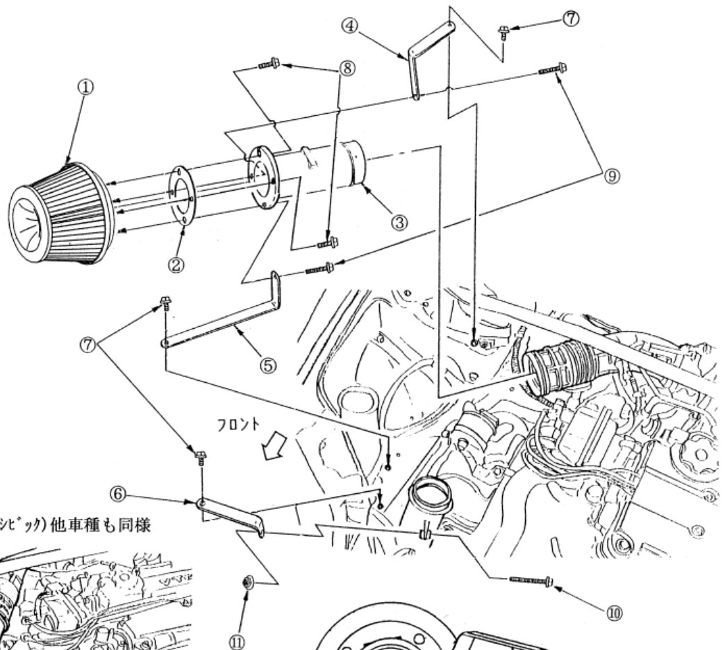
組立図
